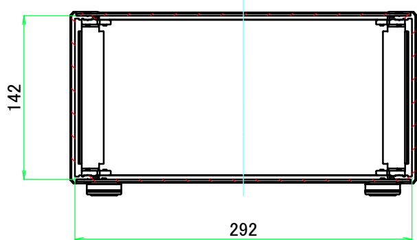
A-A ( 1 : 4.5 )
