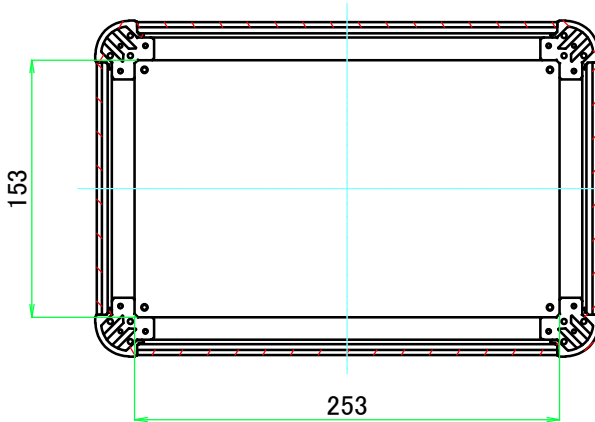
C-C ( 1 : 4.5 )
