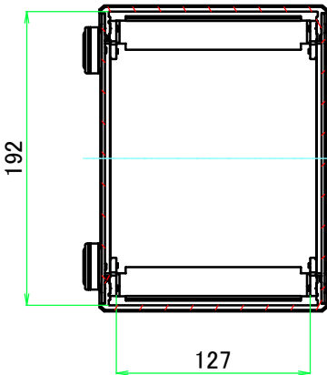
B-B ( 1 : 4.5 )
